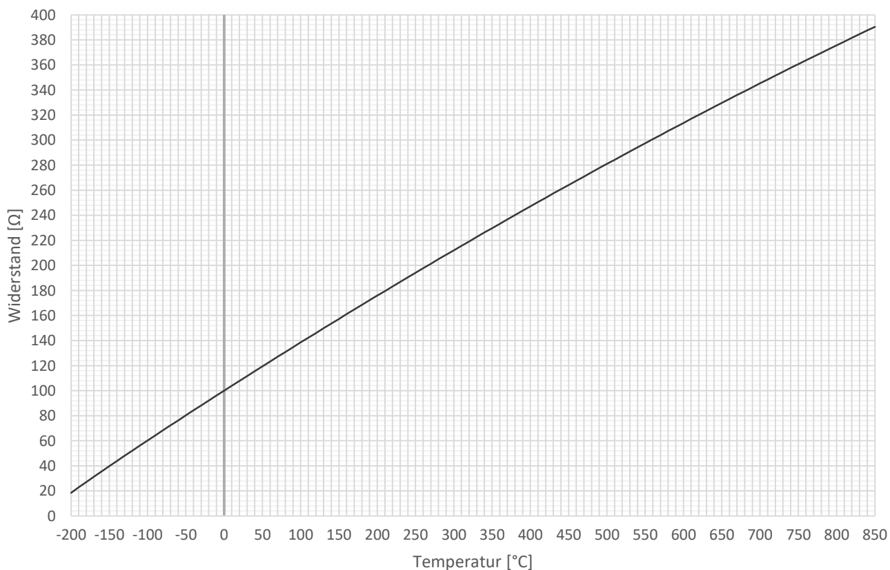
Kennlinie Pt100
